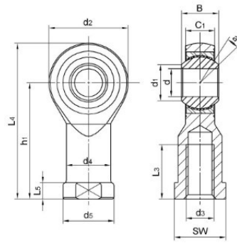
尺寸 mm
