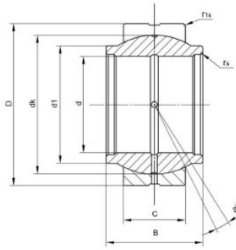
尺寸(mm)
